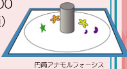
円筒アナモルフォーシス
